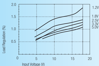
R-53xx / R-54xx Input Voltage Load Regulation VS Vin
